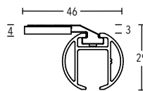
Deckenträger 3 mm Art.-Nr. 702013
