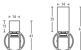
Deckenträger 15 mm Art.-Nr. 702015 + 702035
