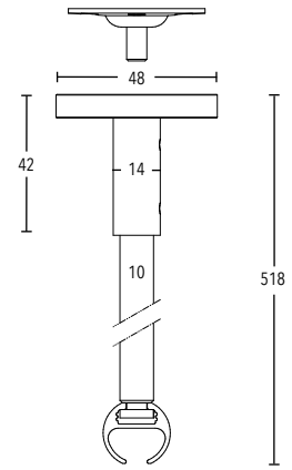
Deckenträger 500 mm Art.-Nr. 702050
